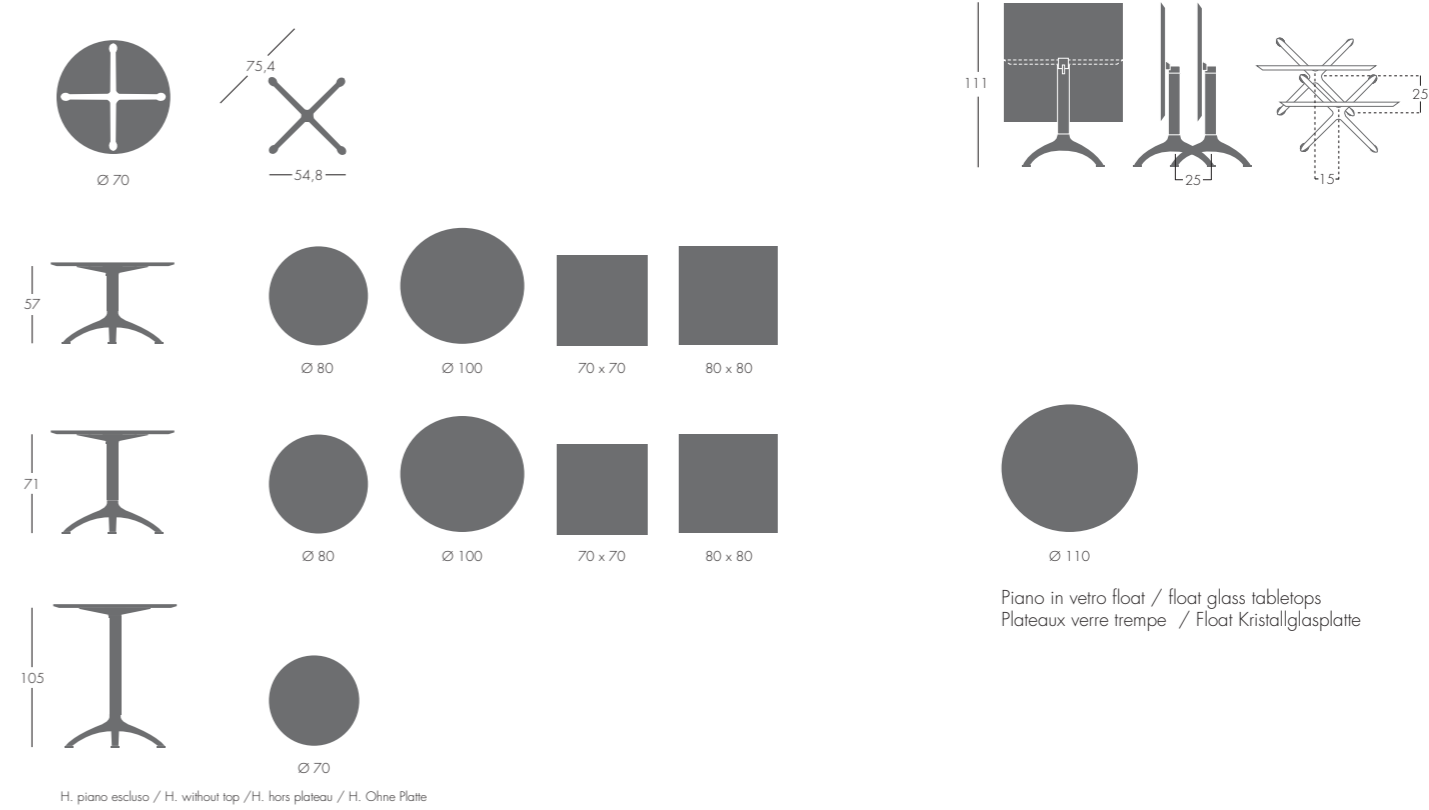
H. piano escluso / H. without top / H. hors plateau / H. Ohne Platte
